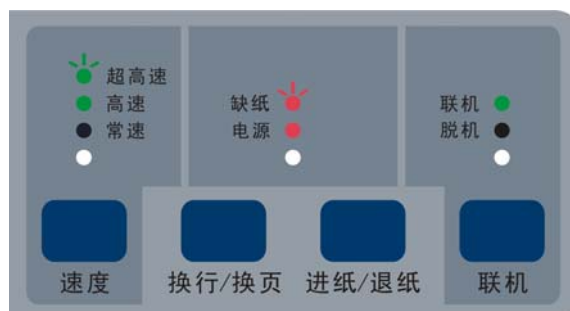
图 4-1 控制面板
