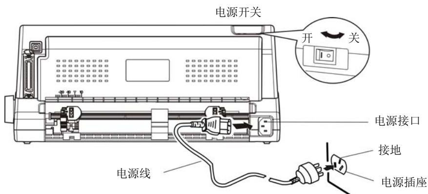
图 2-12 连接电源线
