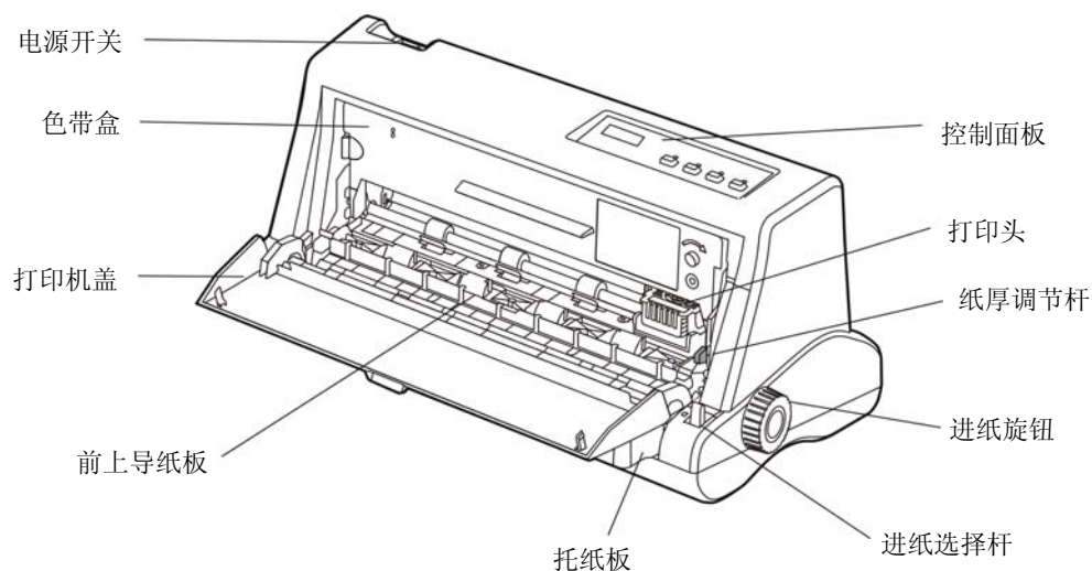
图 2-3 打印机主要部件（前视图）
