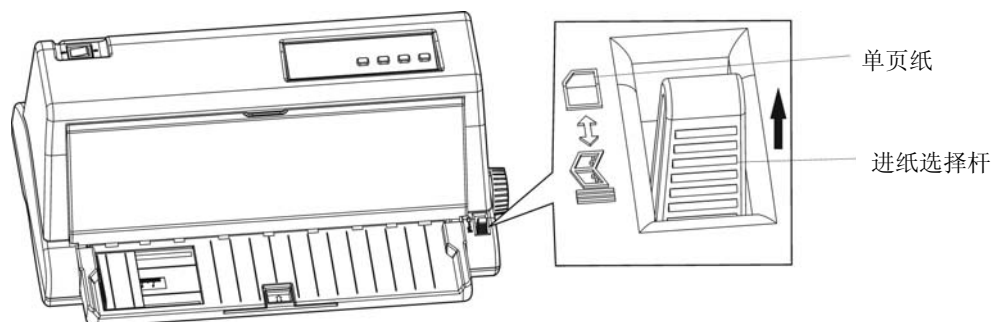
图 3-2 设定进纸位置（单页纸）
