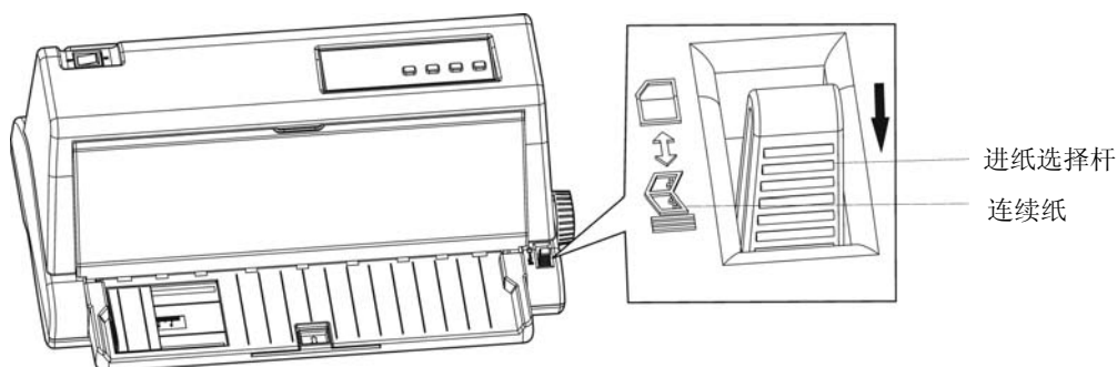
图 3-7 设定进纸选择杆位置（连续纸）
