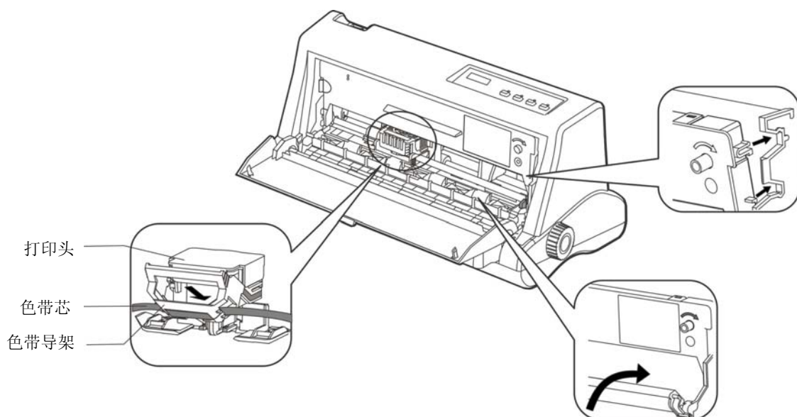
图 2-9 安装色带盒
