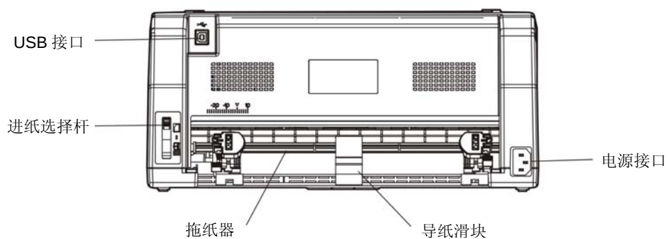
图 2-3 打印机主要部件（后视图）
