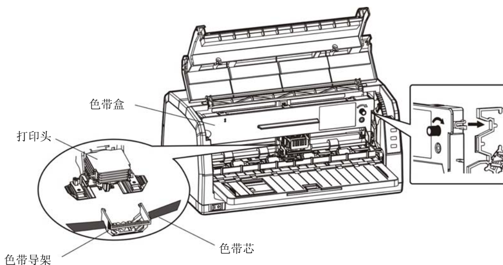
图 2-8 安装色带盒
