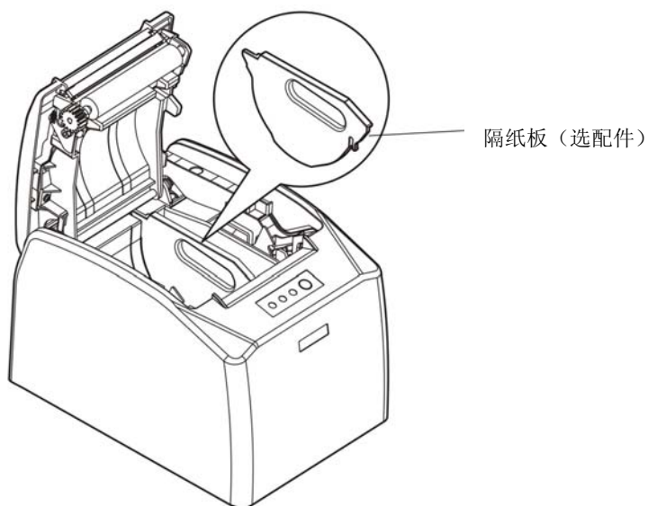
图 4-2 安装隔纸板 (选配件)
