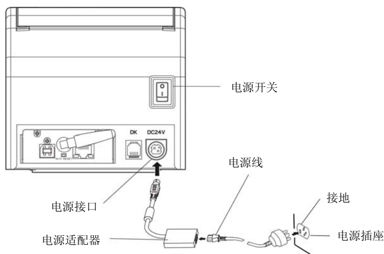
图 2-5 连接电源
