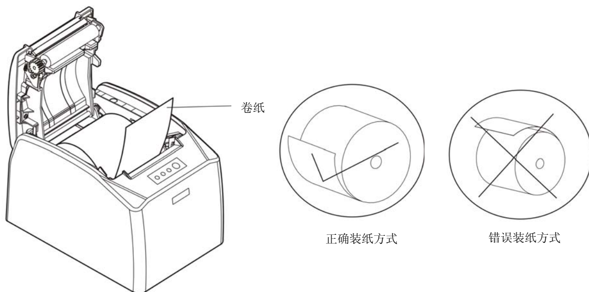
图 4-3 卷纸放进纸斗的方向
