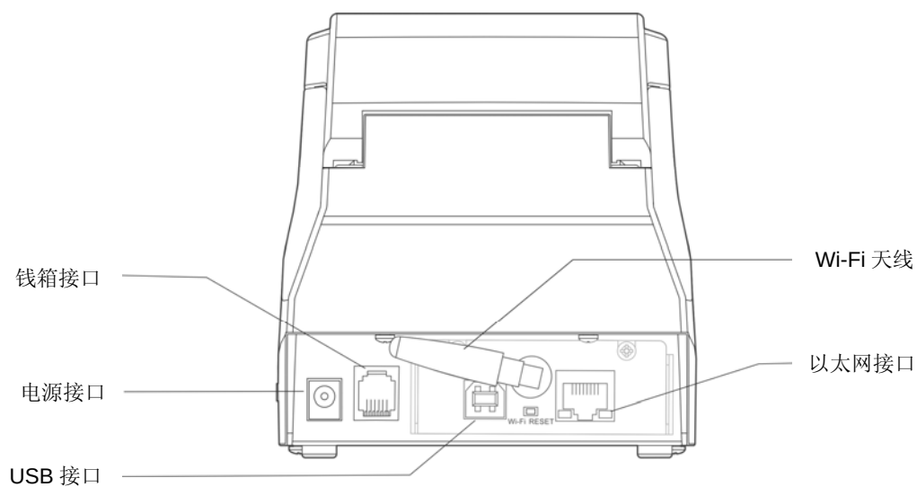
图 1-4 MCP-58GF 打印机背面接口
