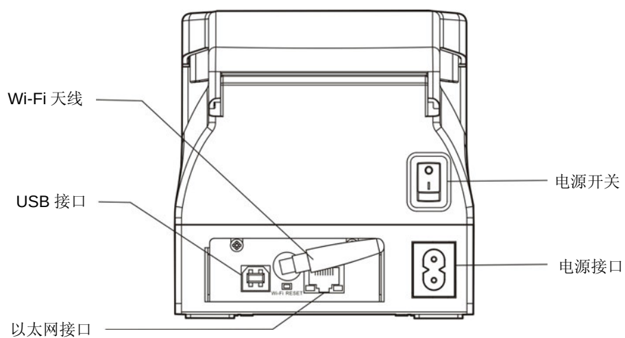
图 1-2 MCP-58 打印机背面接口
