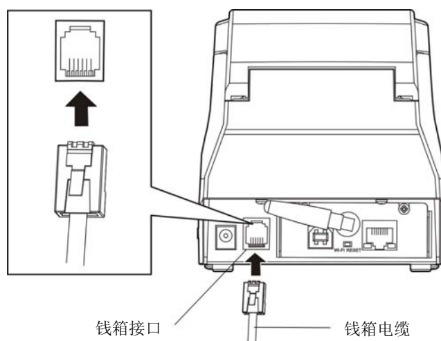
图 2-3 连接钱箱电缆
