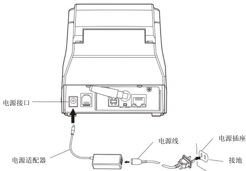
图 2-6（2） MCP-58GF 连接电源
