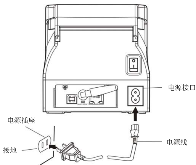
图 2-6 (1) MCP-58 连接电源
